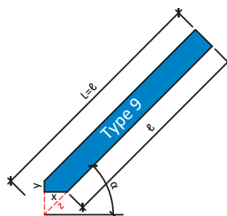
Verticale & horizontale afschuining goot (basisafschuining verticaal => verlenging z) Toegelaten helling 32° tot 58°
